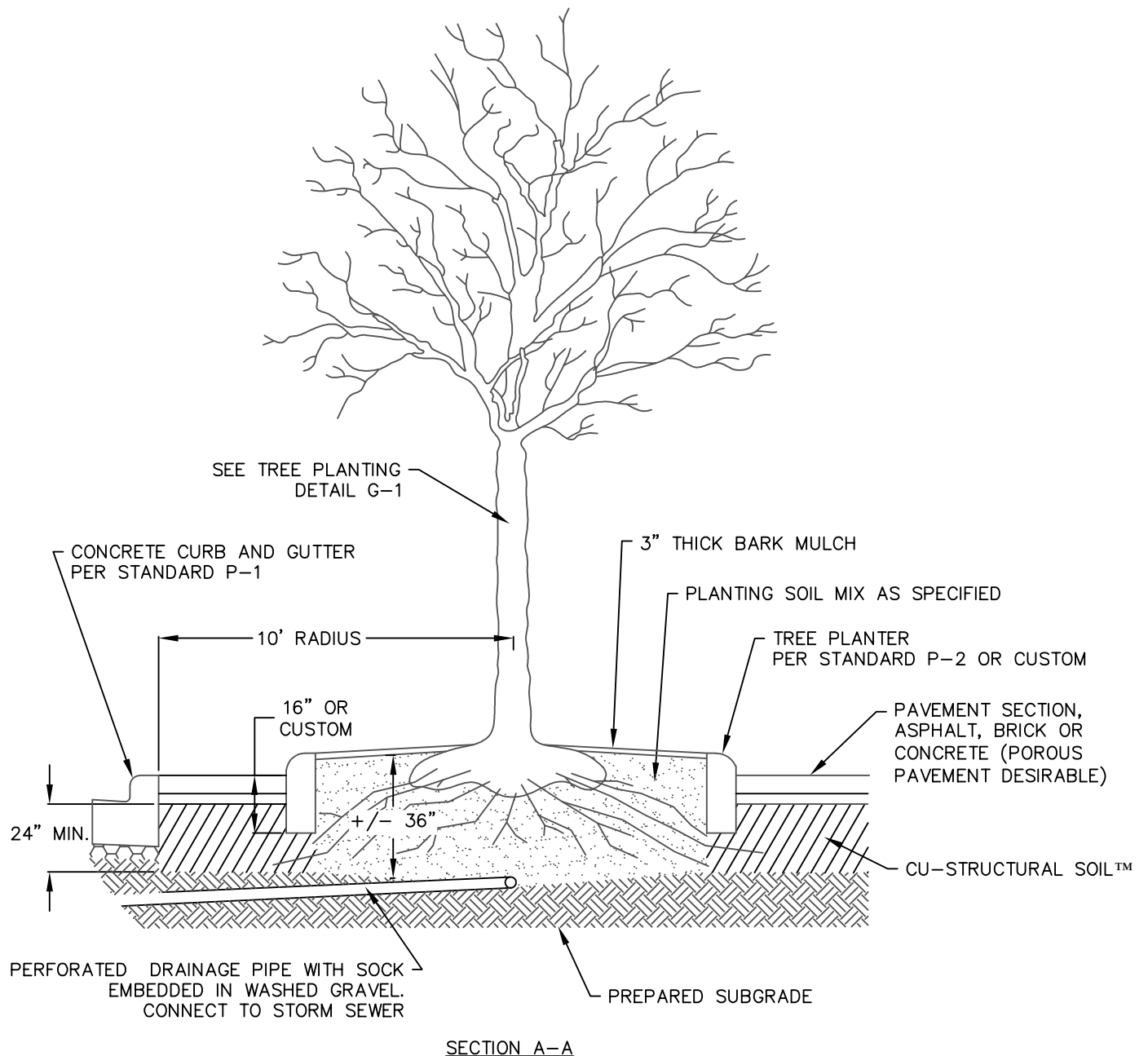
SECTION A-A
